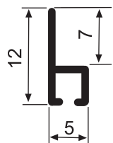
Soporte tipo A
