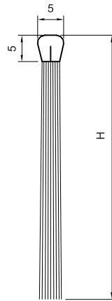
Cepillo Tipo C-5
