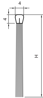
Cepillo Tipo B-4
