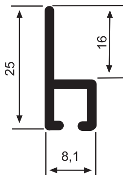
Soporte tipo C
