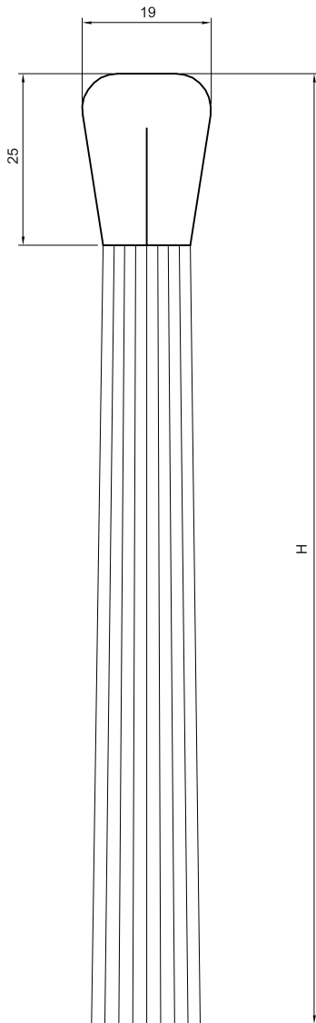
Cepillo Tipo K-19
