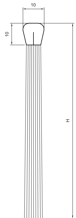
Cepillo Tipo H-10
