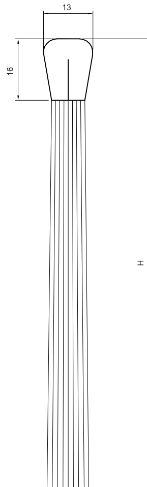
Cepillo Tipo J-13
