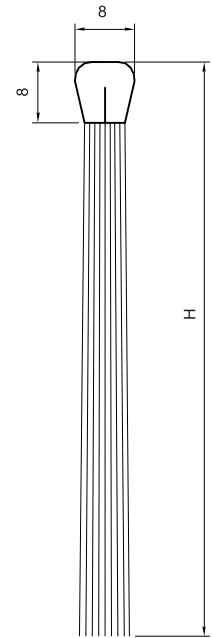
Cepillo Tipo G-8
